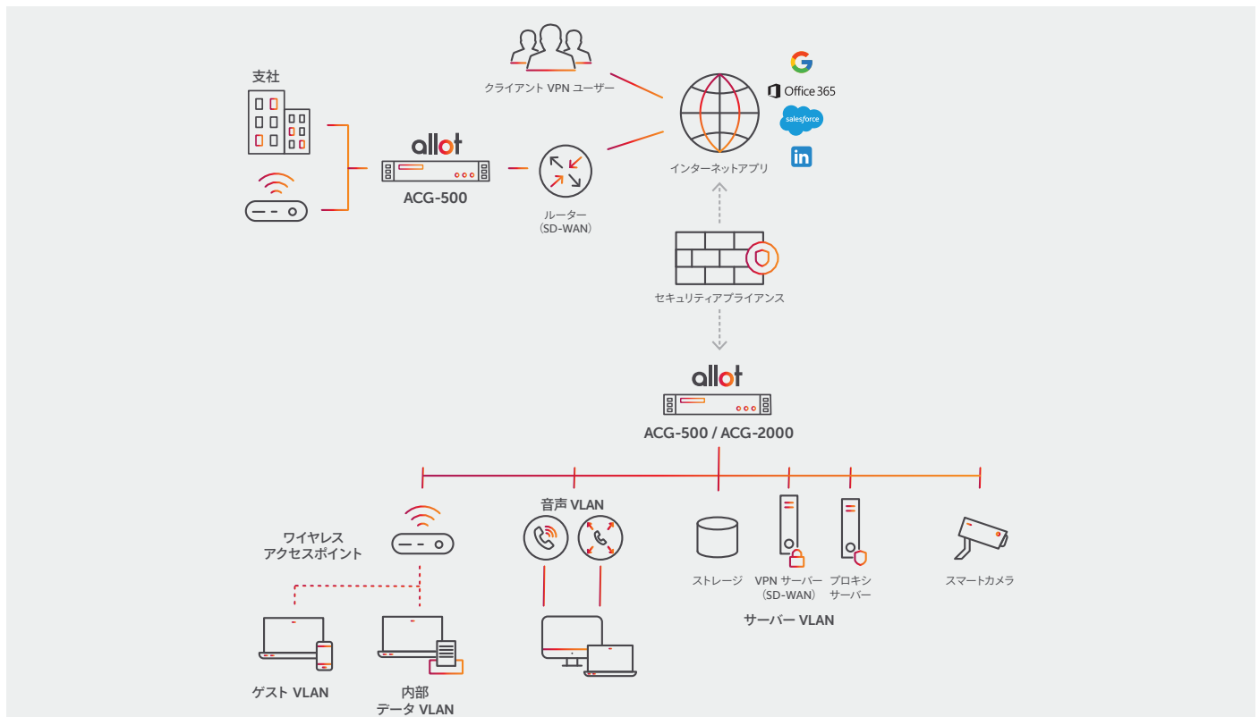
SMB/SME/Enterprise リモートオフィスエコシステムを備えた Allot ACG-500 のアーキテクチャ
